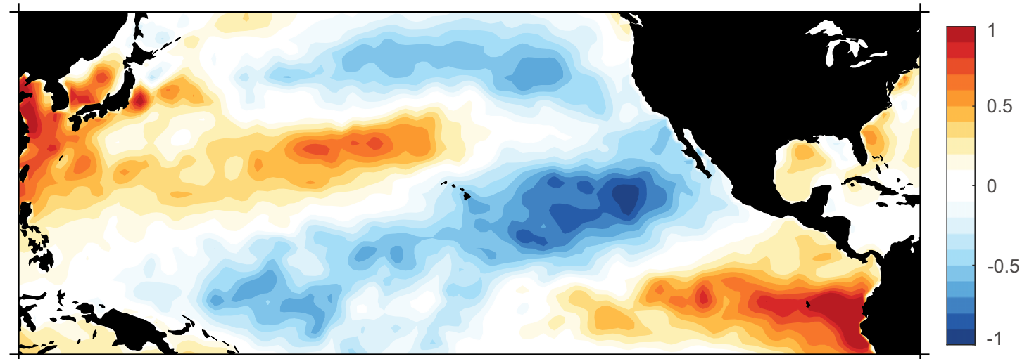
b 1975/1998/1999 Feb-Apr SST anomaly
