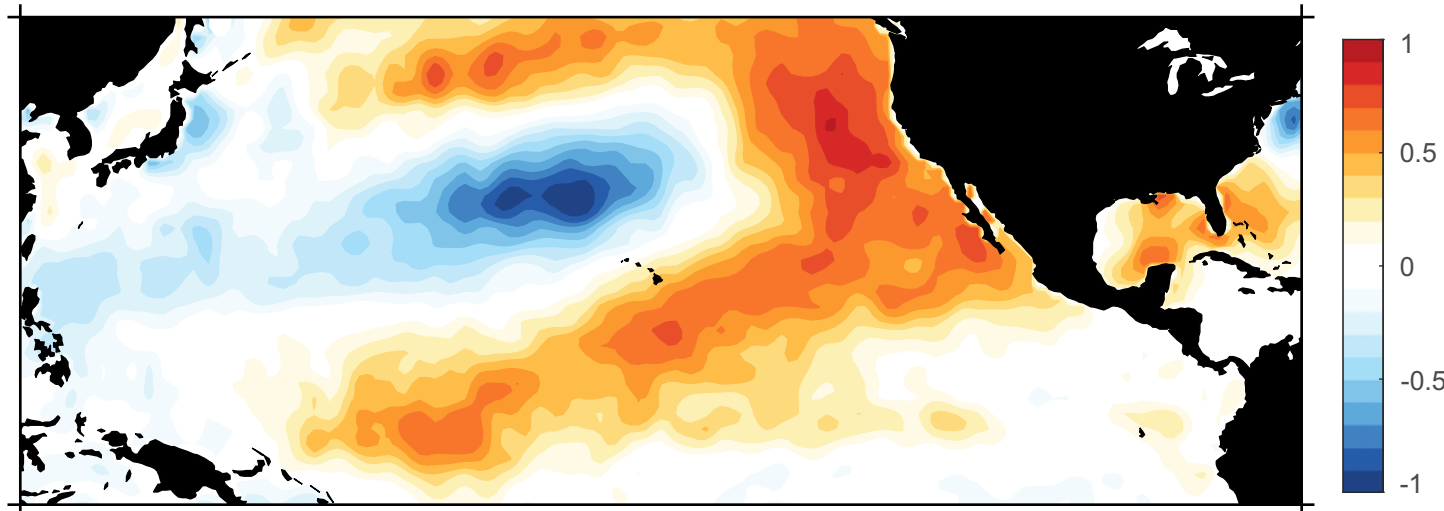
a 1982/1997/2015 Feb-Apr SST anomaly
